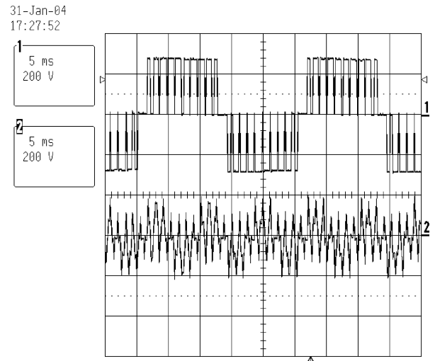
Fig. 12. v_{nm} at F_s = 40 Hz. Ch1: v_{Rn} (Scale: 200 V/div), Ch2: v_{nm} (Scale: 200 V/div).
