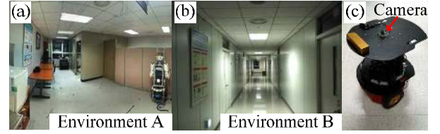
그림 8. 실험환경 및 이동로봇 플랫폼.
