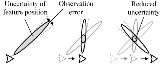
그림 5. 모노카메라 기반 SLAM의 원리.
