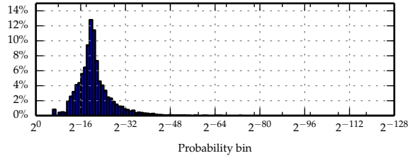
(d) Backoff.
