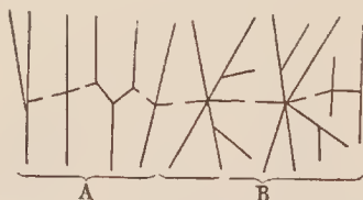
Auflösung der fiederförmigen Gebirgsgliederung.
