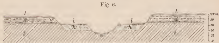
t Tertiär d Decke der diluvialen Nagelfluh h Hochterrassenschotter l Löss n Niederterrassenschotter
