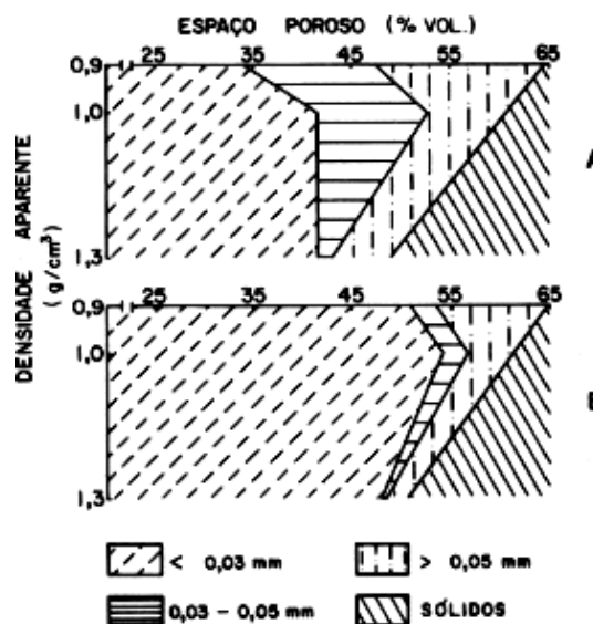
Figura 3. Efeito da densidade aparente na variação do espaço poroso total e na distribuição do tamanho de poros, nos materiais do Latossolo (A) e do Podzólico (B).
