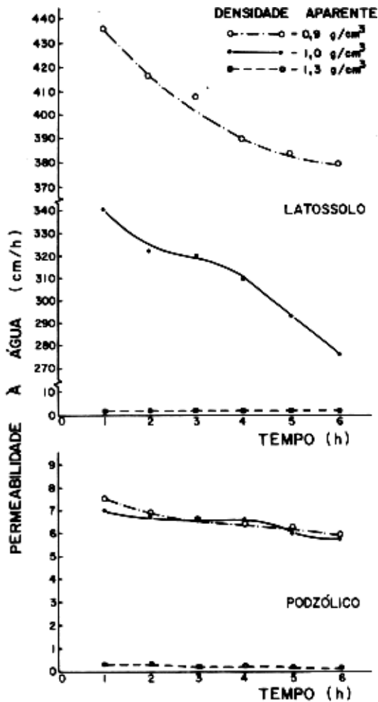
Figura 4. Permeabilidade dos materiais do Latossolo e do Podzólico à água, nas densidades aparentes estudadas.
