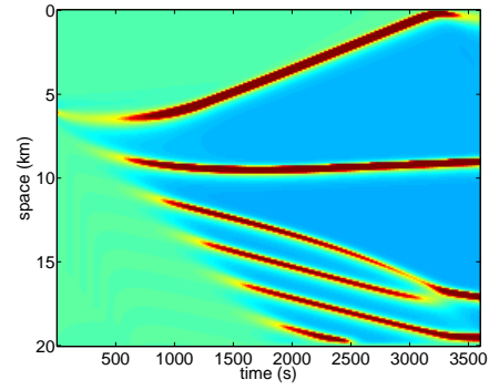
(d) M = 1, \gamma_2 = 0.2, c \neq 0
