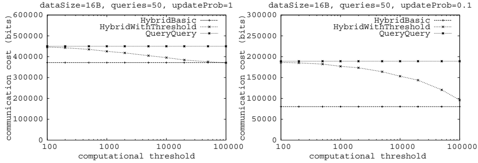
Fig. 5. HybridWithThreshold (D-scenario).
