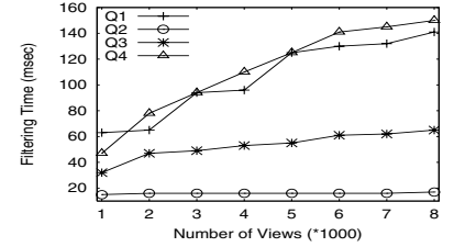
Fig. 12. Filtering Time
