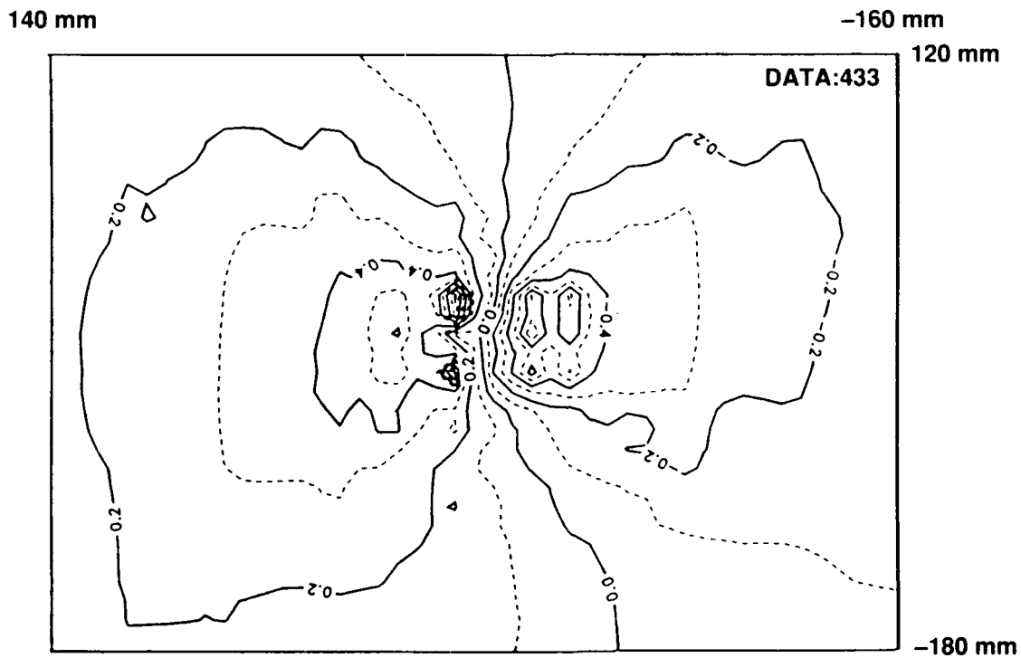
(b) Round-lateral edge
