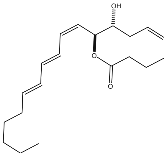
456_neodidemnilactone
