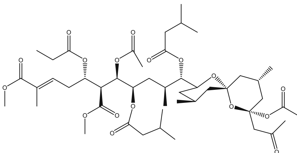
125_Didemnaketals D
