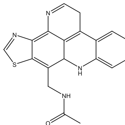
2_Kuanoniamine D
