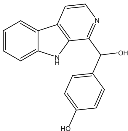
109_Eudistomin Y8
