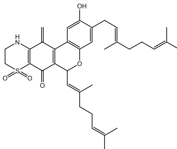
260_thiaplidiaquinones B
