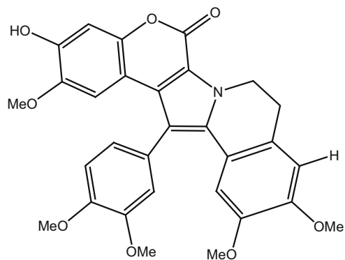
326_lamellarin-J
