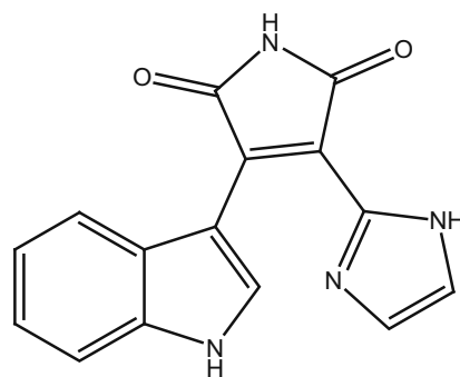
36_neodidemnimide A
