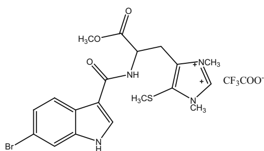
349_leptoclidinamine D
