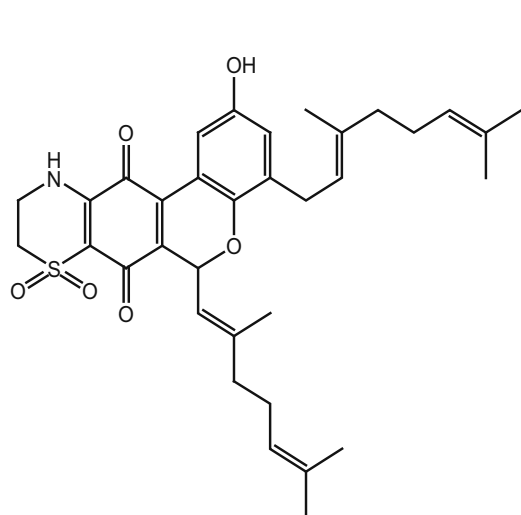
259_thiaplidiaquinones A
