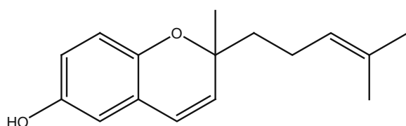
76_Cordiachromene A
