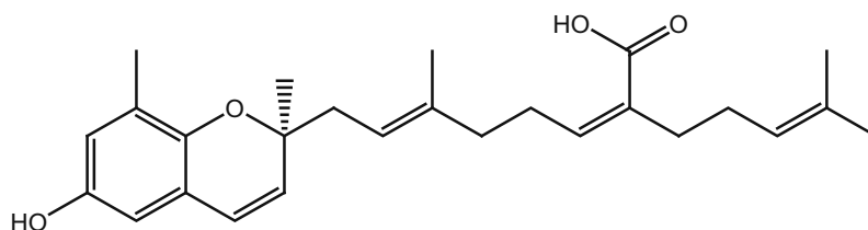
488_(S)-Sargachromenol
