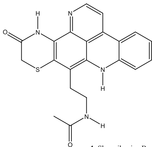
1_Shermilamine B
