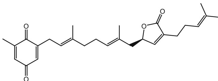
486_yezoquinolide
