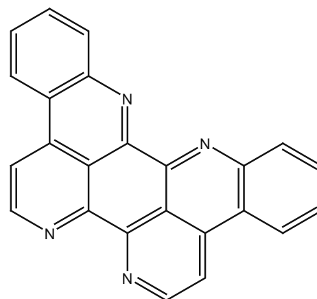
190 eilatin
