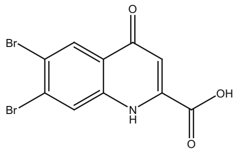
502_Caelestine B
