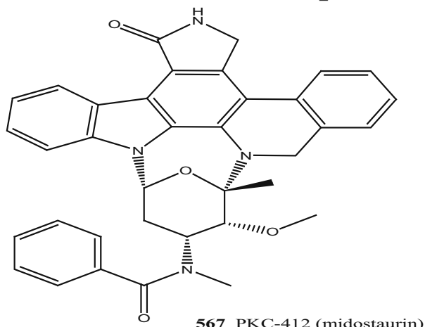
567_PKC-412 (midostaurin)
