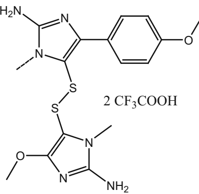
430_polycarpine
