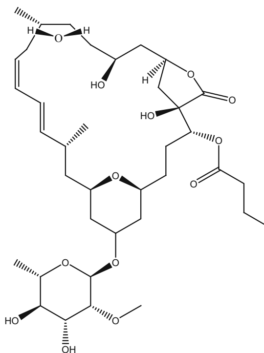
337_mandelalides B
