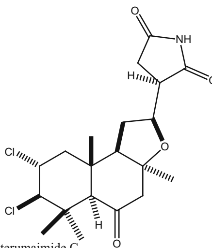
361_haterumaimide C
