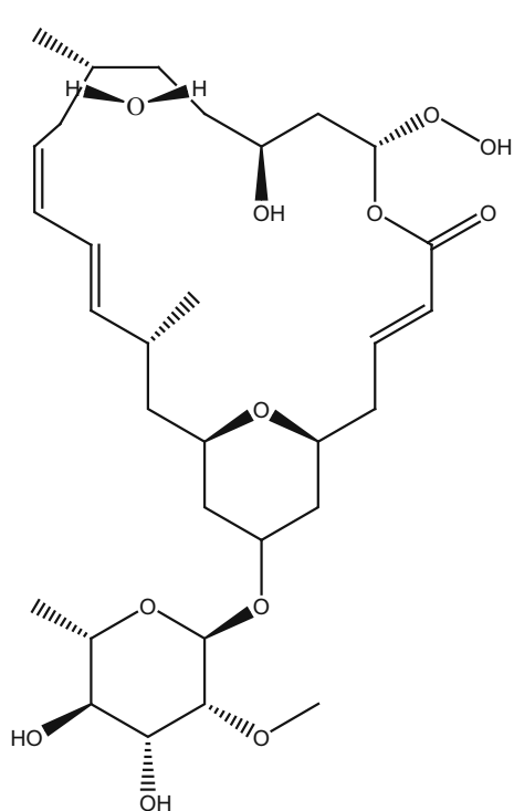
336_mandelalide A
