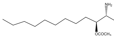
358_clavaminol F
