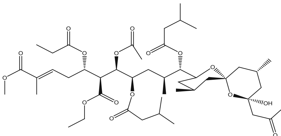
126_Didemnaketals E
