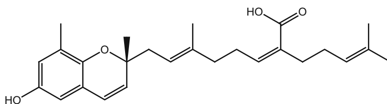
487_(R)-Sargachromenol
