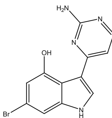
90_Meridianin B
