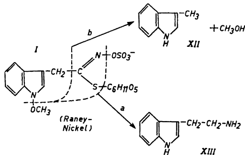
Abb. 4. Hydrogenolytische Spaltung von Neoglucobrassicin.
