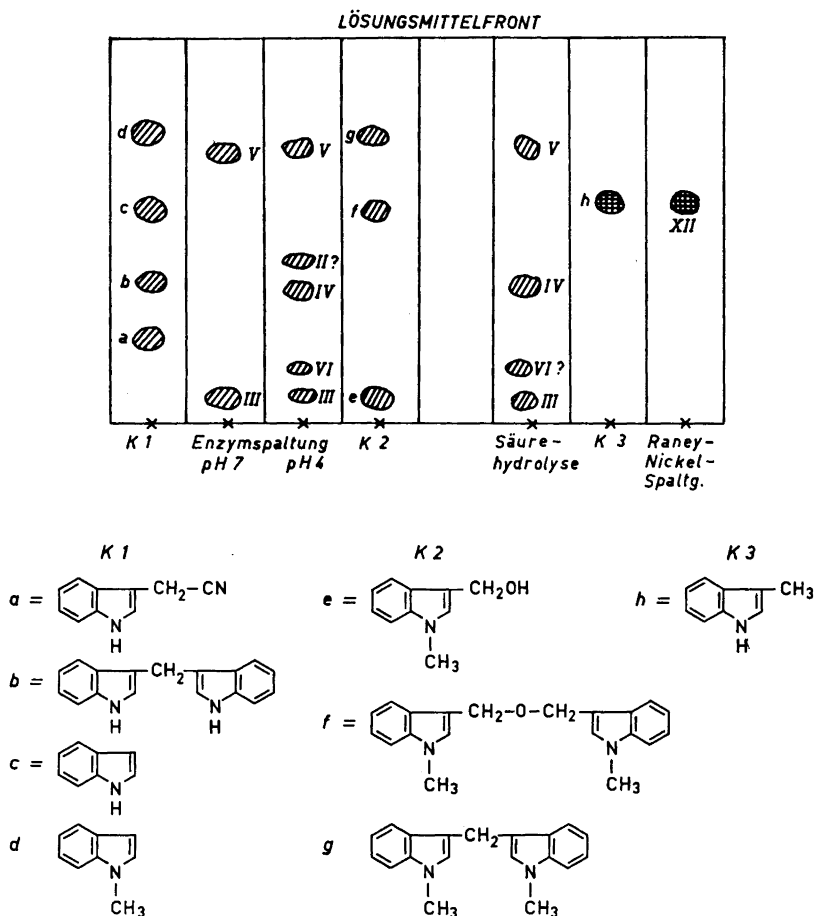
Abb. 5. Dünnschichtchromatogramme von einigen Indolderivaten und Produkten, welche bei der enzymatischen, hydrolytischen und hydrogenolytischen Spaltung von Neoglucobrassicin entstehen. Trägerschicht: Kieselgel G. Fließmittel: Benzol.
