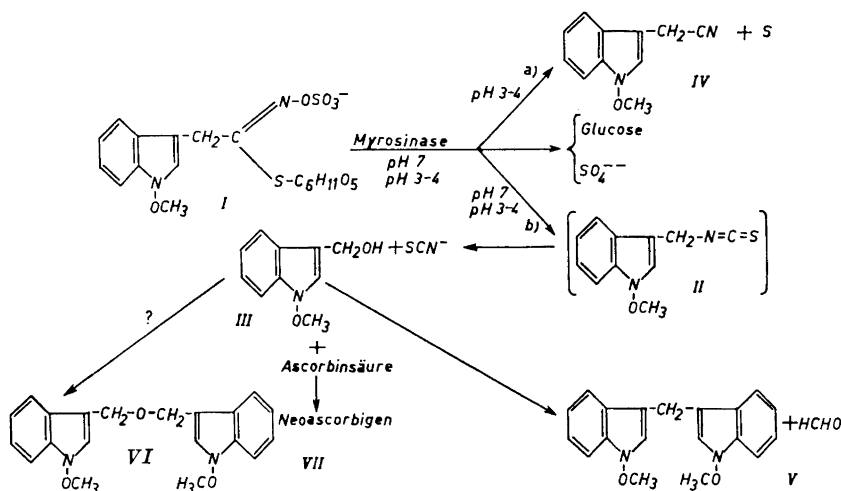
Abb. 2. Enzymatische Spaltung von Neoglucobrassicin und dabei gebildete verschiedene Produkte.
