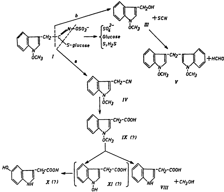
Abb. 3. Hydrolytische Spaltung von Neoglucobrassicin.
