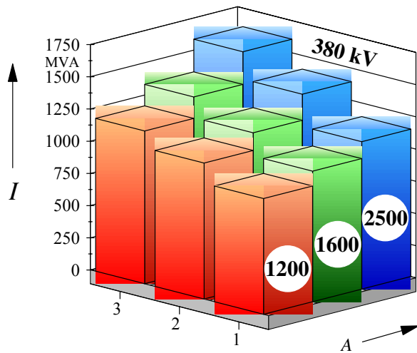
Abb. 7: Übertragungsleistungen von 380 kV-Kabeln unterschiedlicher Kupferleiter-querschnitte und Legenanordnungen
