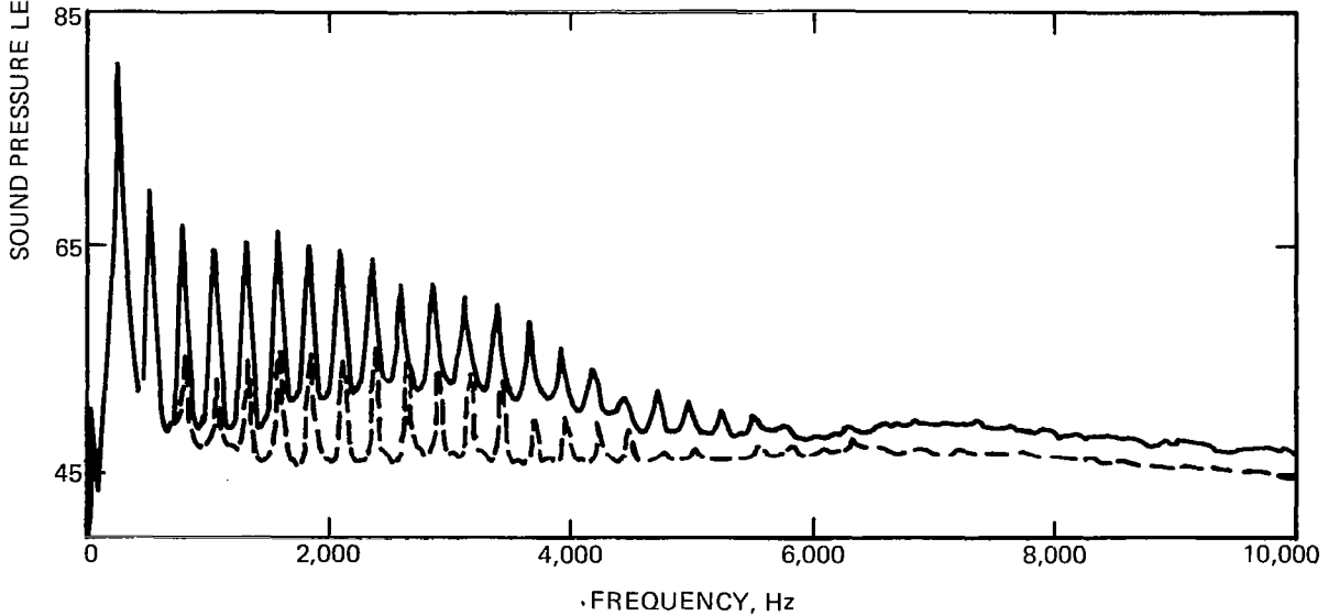
(d) AIRFOIL TIP 15 cm INBOARD OF ROTOR TIP
