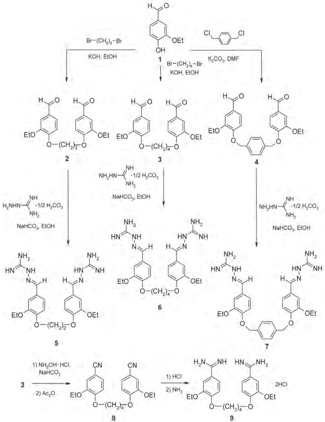
Рис. 3. Схема синтеза исследуемых соединений
