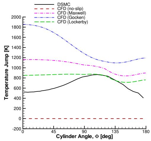
(d) Kn = 0.25
