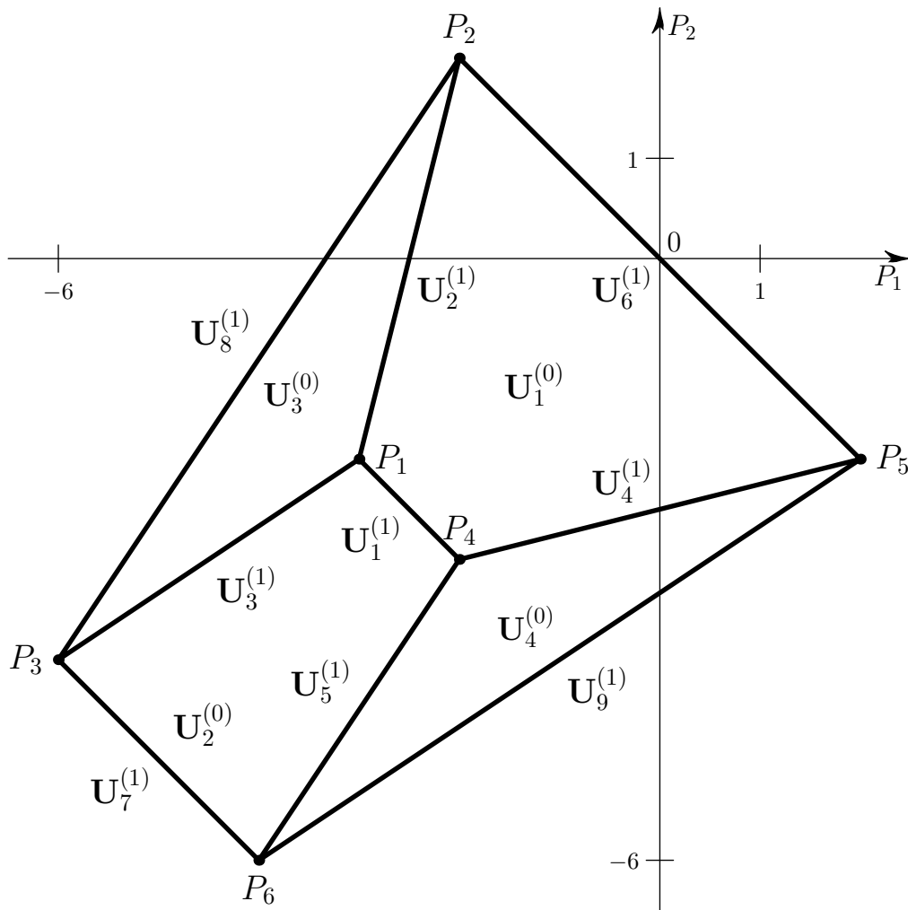
Рис. 2. Концентрированные нормальные конусы \mathring{\mathbf{U}}_j^{(d)} в координатах p_1, p_2 . Верхние кружочки опущены.
