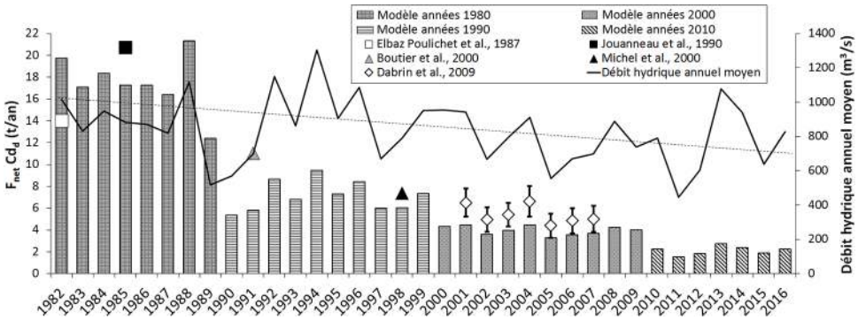
Fig. 7. Les barres grisées et hachurées donnent les variations interannuelles et inter-décennales des flux nets de Cd_d en tonne/an. La variation interannuelle des flux hydriques en m^3/s est également reportée. Les figurés blancs, noirs et gris correspondent aux valeurs des flux nets publiés antérieurement.
