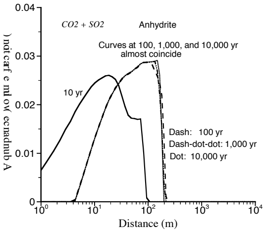
(a) Anhydrite
