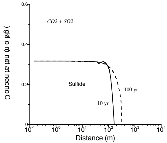
(b) Sulfide
