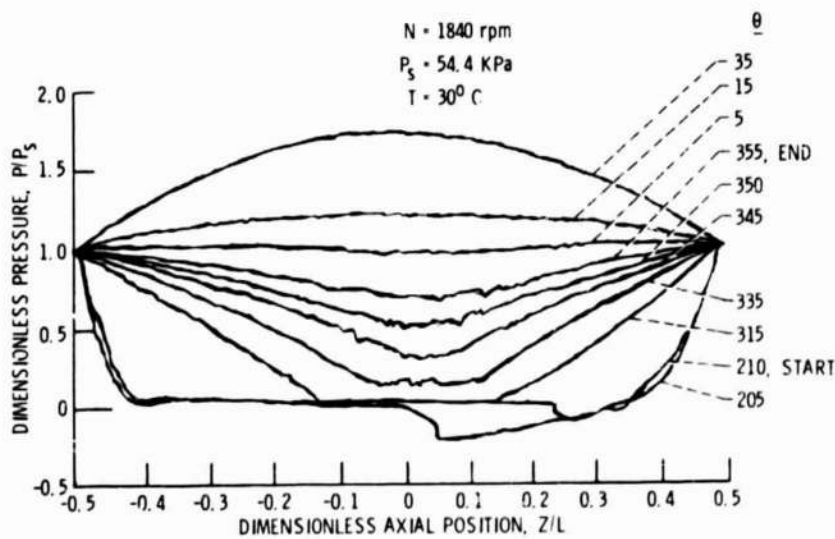
(d) N = 1840 \text{ rpm} ; P_s = 54.4 \text{ KPa} .
