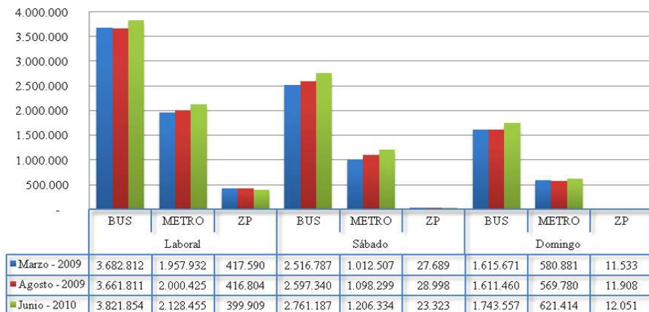
FIGURA 3: Transacciones por Tipo de Operador y Día
