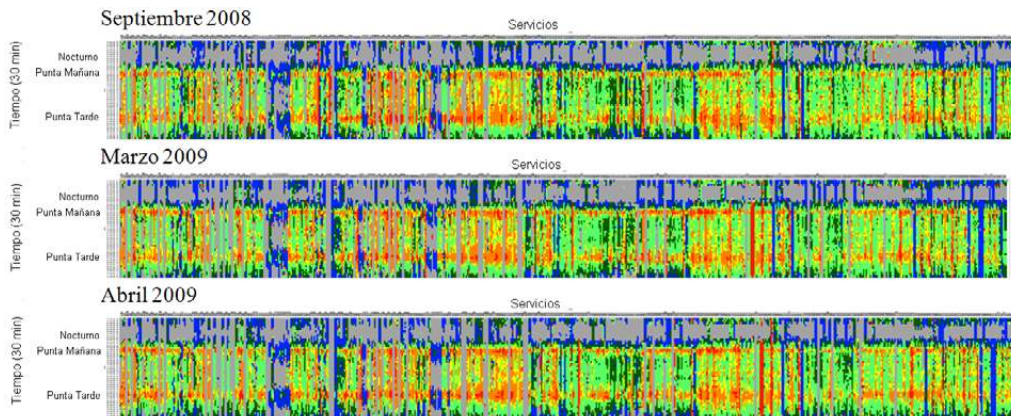
FIGURA 13: Velocidades Comerciales de Todos los Servicios cada Media Hora
