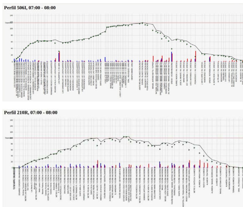
FIGURA 18: Ejemplos de Perfiles de Carga de por Servicio (pasajeros que validan)
