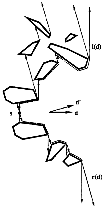
Figure 4.2. Sweeping the paths l(d) and r(d) .
