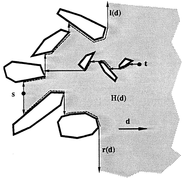
Figure 4.1. Defining l(d) , r(d) , H(d) , waterfall paths.
