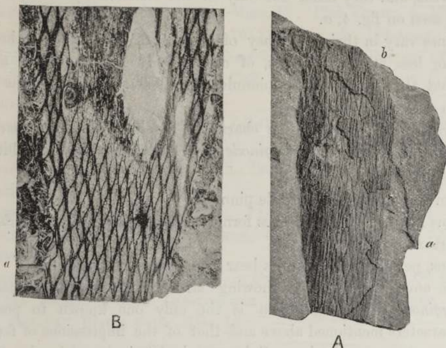
FIG. 5.— Crossothea Höninghausi , BRONGT. sp. ( Lyginodendron Oldhamium , WILL.).
