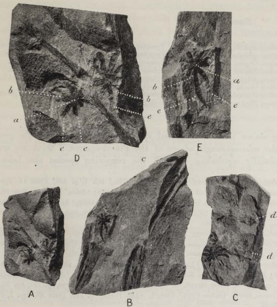
FIG. 11.— Diplothea stellata , KIDSTON.
