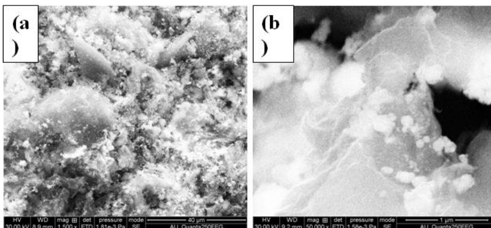
Fig.4. (a,b) SEM images of Ag-RGO nanocomposite.
