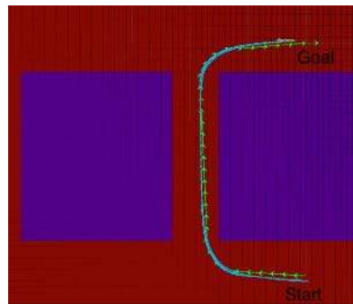
(d) RRT* with Dubins: Query 2
