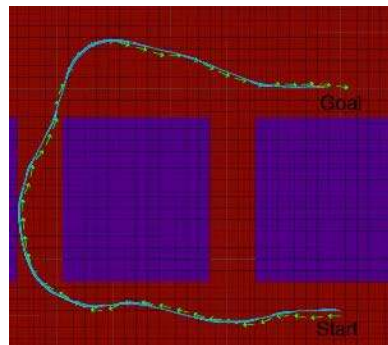
(b) RRT: Query 2
