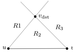
FIG. 2.5. The proof of Lemma 2.2.
