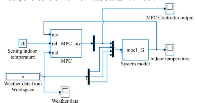
Fig. 6. MPC controller.
