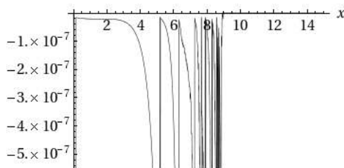
FIG. 15. TV(x; b^*) - V(x; b^*)
