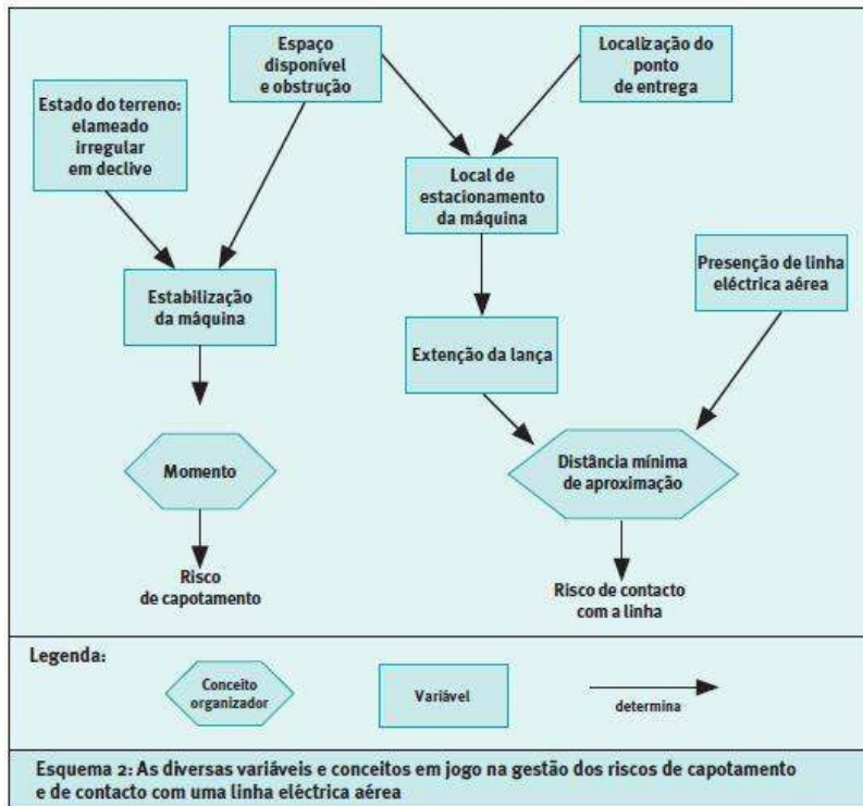
Esquema 2 : As diversas variáveis e conceitos em jogo na gestão dos riscos de capotamento e de contacto com uma linha eléctrica aérea
