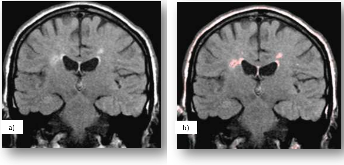
Figura 56 - Imagem ponderada em T2 com FLAIR, em orientação coronal da região do corpo caloso. a) Imagem original; b) Imagem após aplicação da GUIAL para reconhecimento das HSB, assinaladas a vermelho. (Fonte: Autor)
