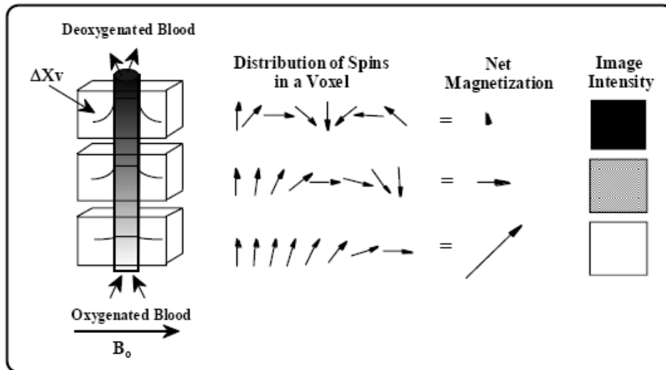
Figura 26 - Esquema da passagem do sangue de oxigênio para desoxihemoglobina e o correspondente efeito sobre a fase dos spins. (Fonte: Shetty, N. et al. 2006) (117)
