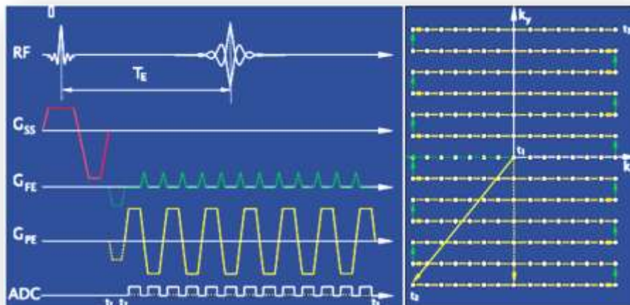
Figura 32 - Diagrama da Sequência EPI e modo “blipped” de preenchimento do Espaço K . (Baert, A., 2005). (216)
