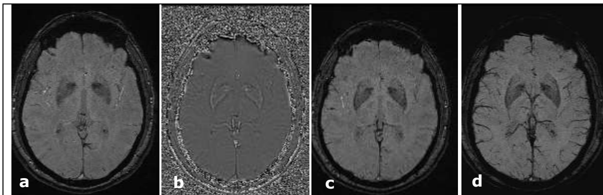
Figura 45 - Imagens obtidas pela técnica SWI. a - Imagem de magnitude; b - Imagem de fase; c - Imagem SWI; d - Imagem de minIP. (Fonte: Autor)
