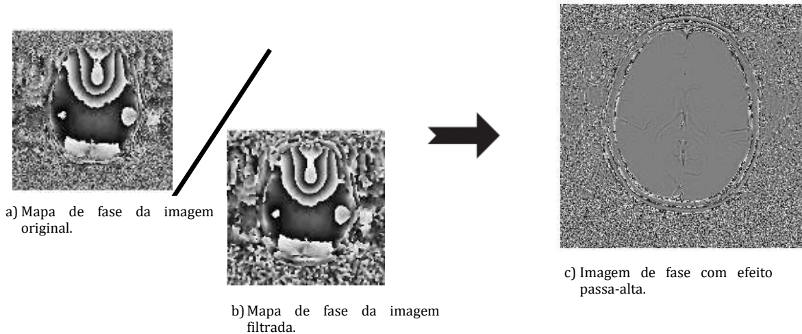
Figura 33 - Esquema representativo da obtenção da imagem de fase corrigida. (Fonte: Haacke, M. 2004). (218)
