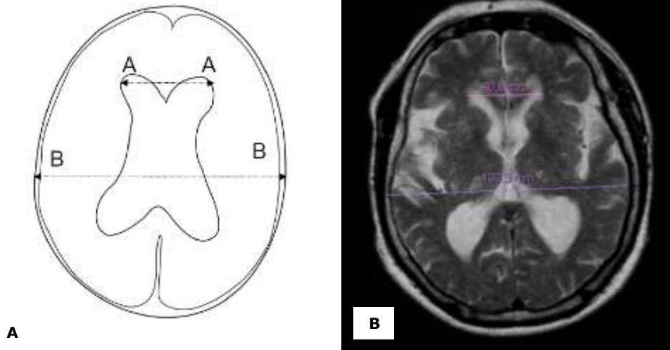
Figura 41 - Metodologia de determinação do índice de Evan ( I = \frac{AA'}{BB'} ) ao nível do plano de Flechsigs . A) Representação esquemática (Fonte: Moore, D. 2012) (109). B) Exemplificação da medição (Fonte: Autor)
