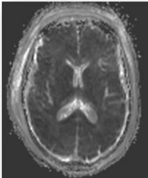
Figura 20 - Imagem do caso 155 pm , em plano axial utilizada para quantificação do ADC nas regiões FC e talâmica. (TR 3200ms; TE 90ms; N.º. de aquisições-1; FA - 90º; espessura de corte 5mm; Mx de Resolução 128x128; intervalo entre cortes 6,75 mm e fator b - de b0 a b1000 ). (Fonte: Autor)
