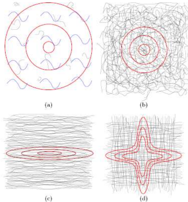
Figura 28 - Esquemas representativos da iso e anisotropia na difusão das moléculas de água de acordo com a cito-arquitetura do cérebro. As linhas a negro representam as barreiras impostas ao movimento das moléculas de água, as linhas vermelhas correspondem à probabilidade p de deslocação, ou movimento esperado, em cada tipo de constituinte cerebral. a) Região preenchida por fluido; b) Substância cinzenta isotrópica; c) e d) imagens da SB condicionada a anisotropia numa direção c) e em mais do que uma direção d). (Fonte: Alexander, D. 2007) (200)
