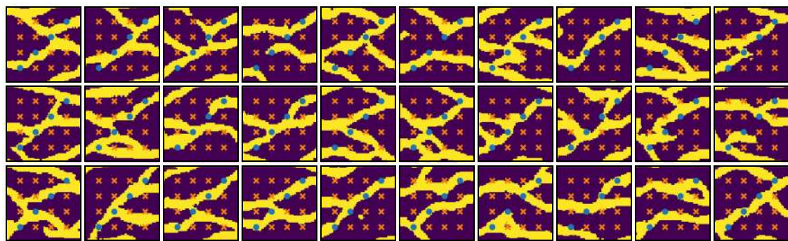
(b) snesim
