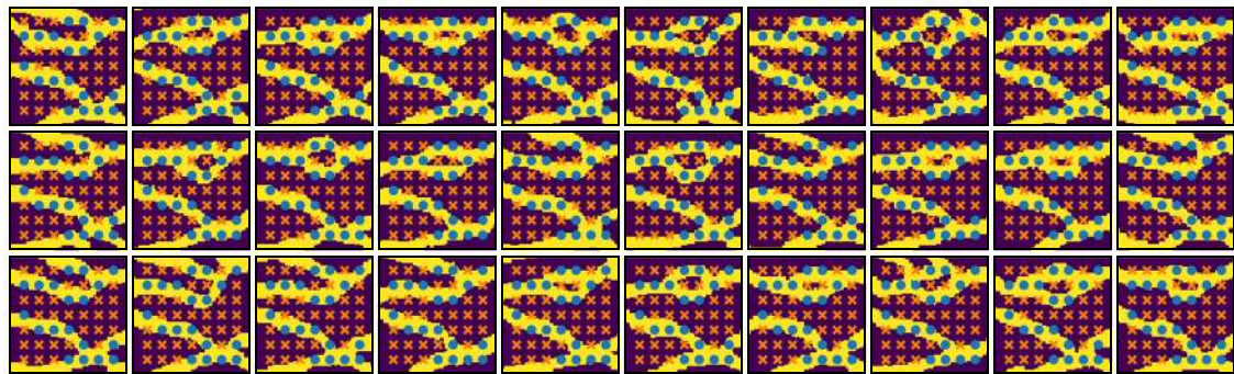
(b) snesim
