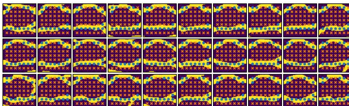
(b) snesim
