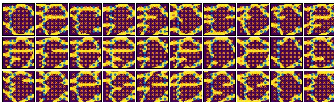
(b) snesim
