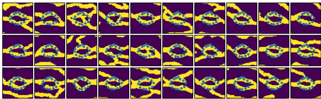
(b) snesim
