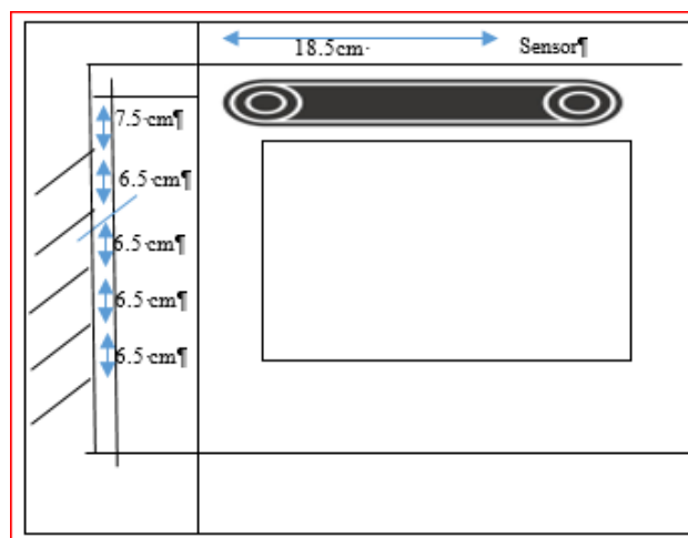
Gambar 2 Desain Mekanik Sistem
