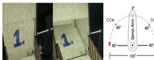
Gambar 6. Sudut Motor Servo Pada Gate
