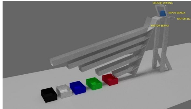
Gambar 3 Visualisasi Desain Mekanik Sistem
