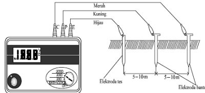
Gambar. 3. Skematik pemasangan elektroda pentanahan dan elektroda bantu untuk proses pengukuran tahanan tanah. (Diambil dari Manual Instruction : Digital Earth Tester 4105 A )
