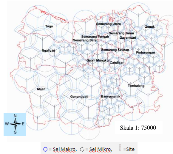
Gambar 8. Hasil rancangan ulang site jaringan radio GSM di kota Semarang.
