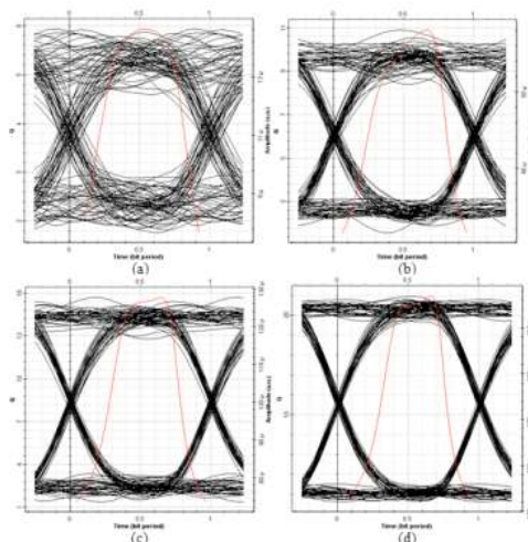
Fig. 5 Diagram for (a) 1TX/1RX (b) 2TX/2RX (c) 3TX/3RX (d) 4TX/4RX.
