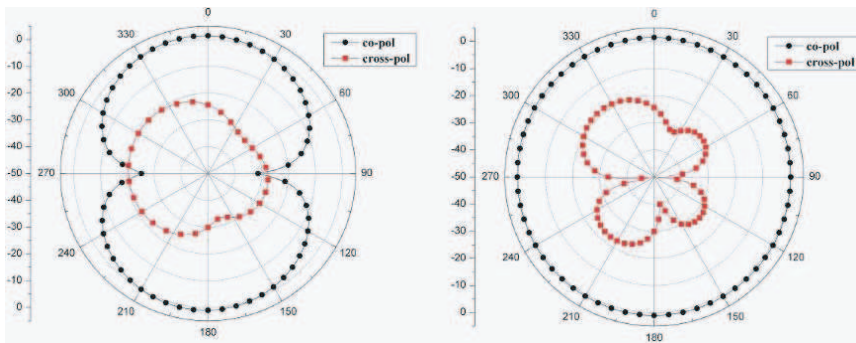
E-plane
