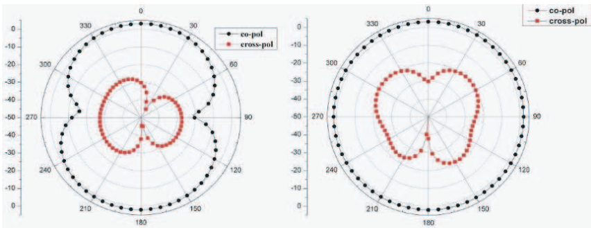
E-plane
