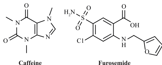
Caffeine
