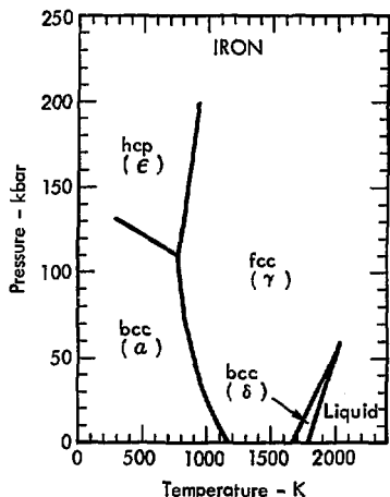
Fig. 28. The phase diagram of iron.
