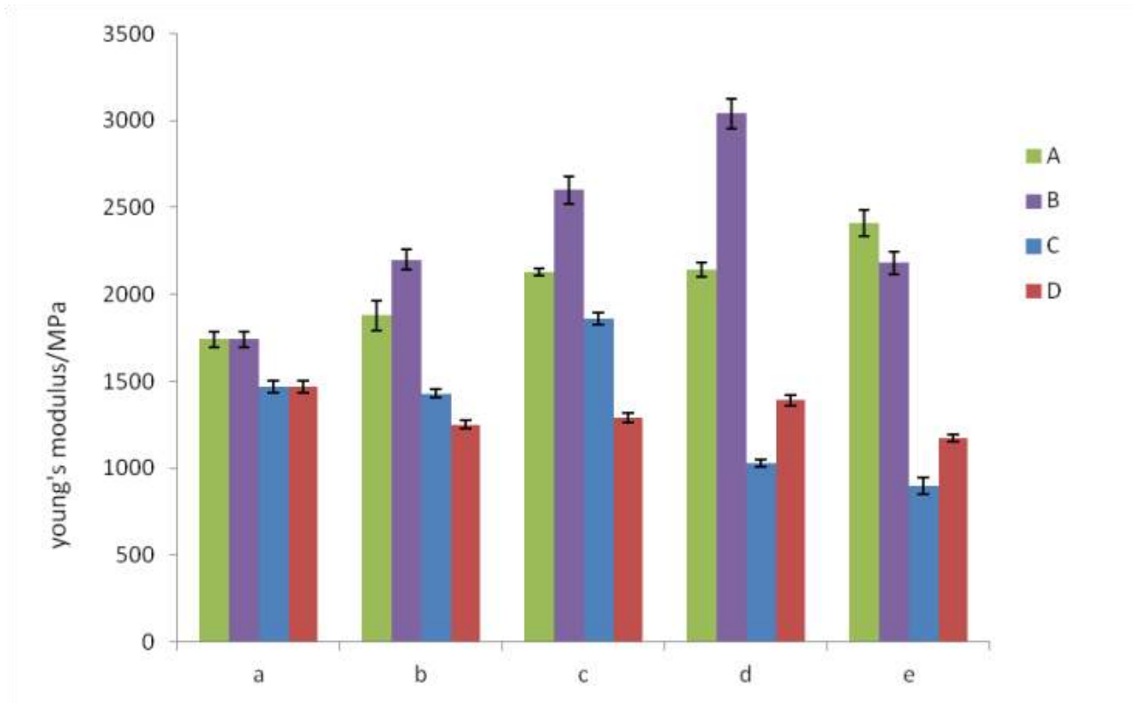
Figure 4.14. The comparison of Young's modulus of polyurethane films before UV irradiation (365nm, 36W, 120h) (A) SiO 2 -TiO 2 nanofibers. (a) blank. (b) F0. (c) F1. (d) F2. (e) F3. (B) SiO 2 -TiO 2 nanotubes. (a) blank. (b) T0. (c) T1. (d) T2. (e) T3. After UV irradiation (365nm, 36W, 120h) (C) SiO 2 -TiO 2 nanofibers. (a) blank. (b) F0. (c) F1. (d) F2. (e) F3. (D) SiO 2 -TiO 2 nanotubes. (a) blank. (b) T0. (c) T1. (d) T2. (e) T3.
