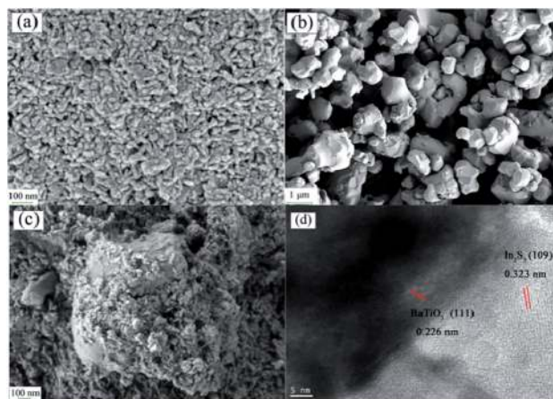
Fig. 2 SEM images of (a) IS, (b) pristine BT, (c) BTIS, and HRTEM image of (d) BTIS.
