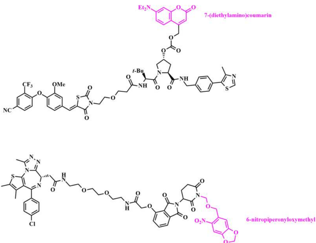
Figure 7. Chemical structures of DEACM- and NPOM-containing pc-PROTACs Slika 7. Hemijske strukture pc-PROTAC molekula koji sadrže DEACM i NPOM
