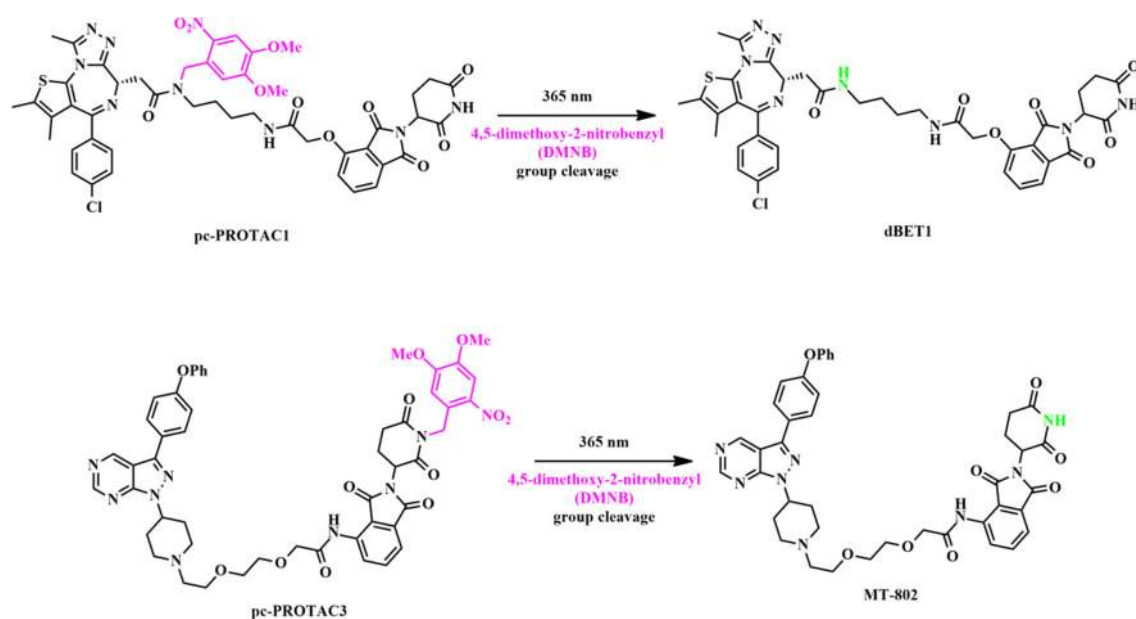
Figure 6. DMNB group cleavage reactions Slika 6. Reakcije uklanjanja DMNB grupe
