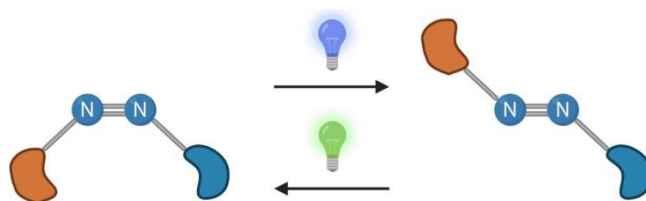
Figure 8. Photoinduced switching between Z - and E -photoPROTAC isomer Slika 8. Fotoindukovani prelaz između Z - i E -photoPROTAC izomera
