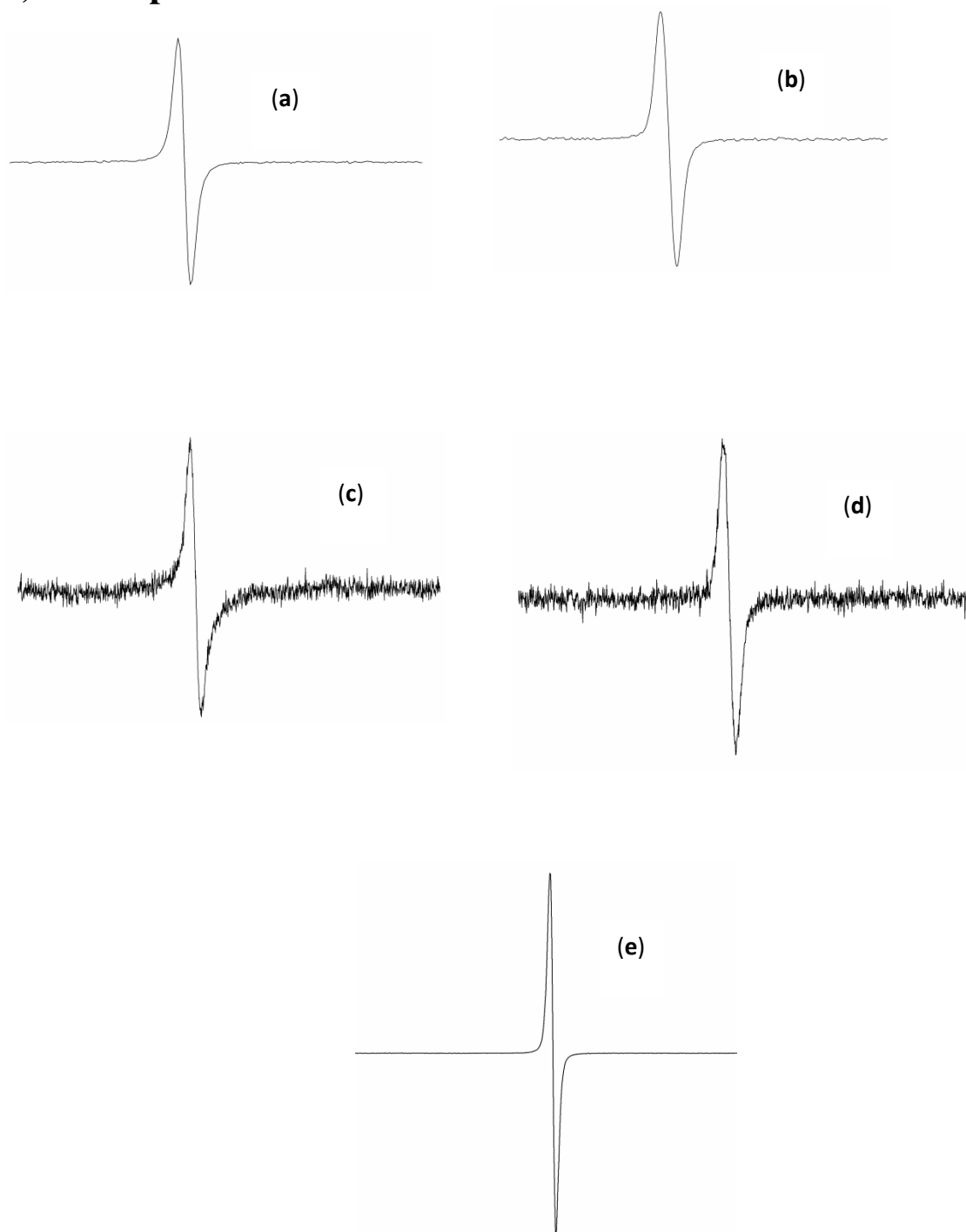
Figure S8. X-band EPR spectra of 1^{+} ( 10^{-3} M) recorded at: (a) 293 K. (b) 167 K. (c) 8 K. (d) 8 K ( 10^{-5} M) (e) 293 K (after 5 equiv oxidant)
