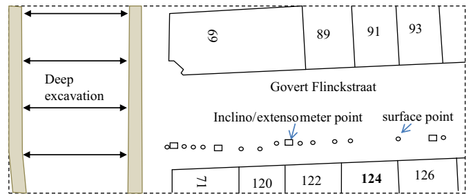
Fig. 15. Top view of deep excavation and buildings Govert Flinkckstraat (Ceintuurbaan)
