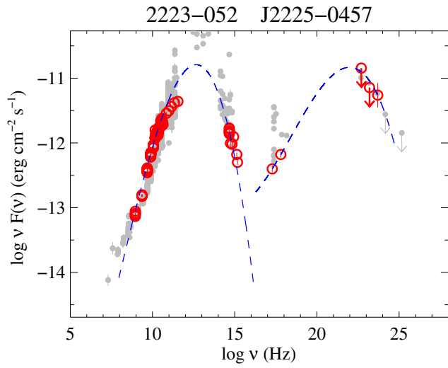
Fig. 115. 2223-052.
