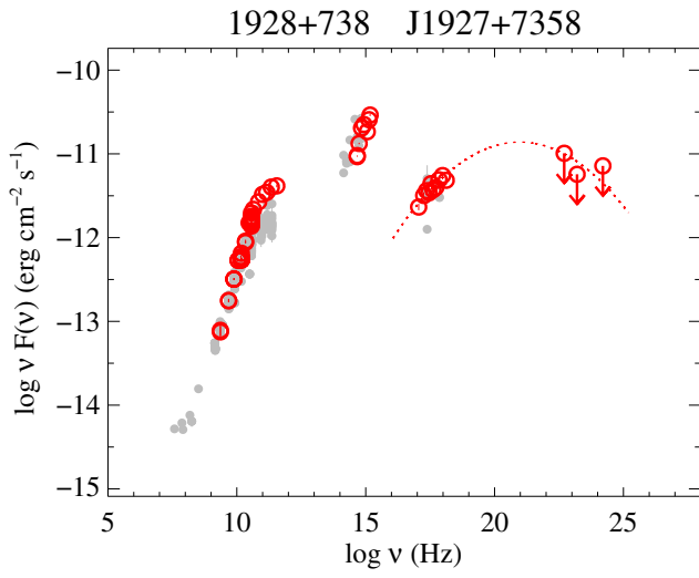
Fig. 100. 1928+738.
