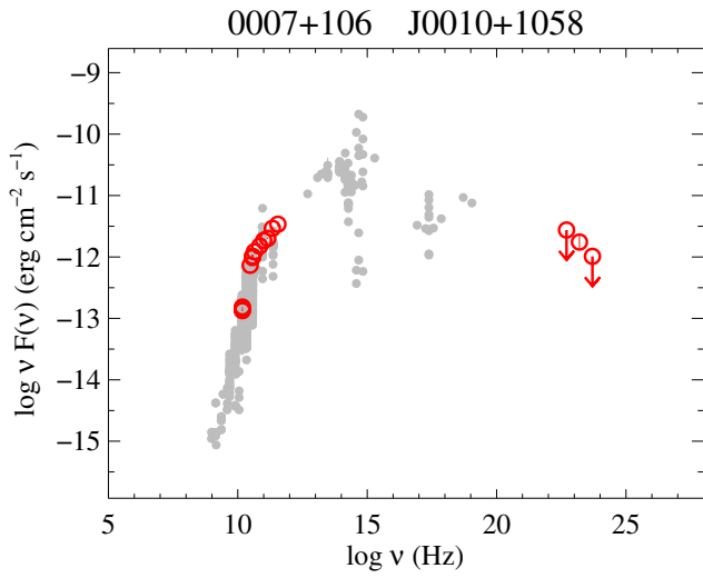
Fig. 19. 0007+106.
