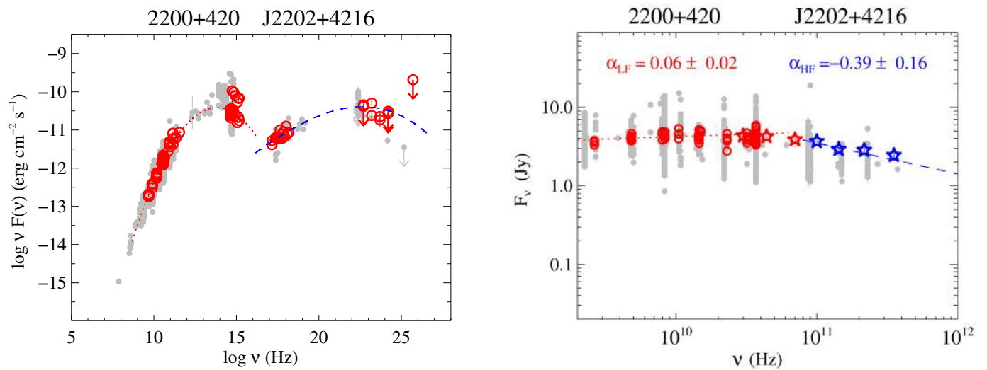
Fig. 111. 2200+420.
