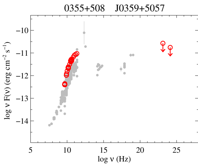
Fig. 36. 0355+508.
