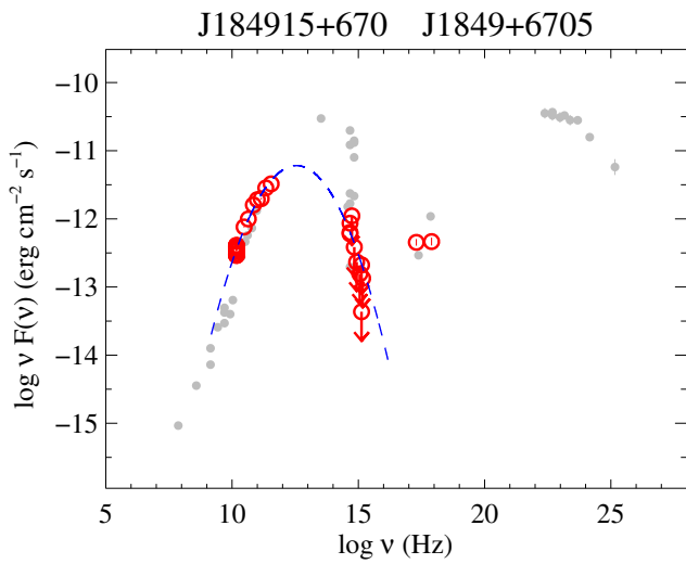
Fig. 99. J184915+670.
