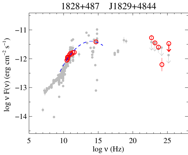
Fig. 98. 1828+487.
