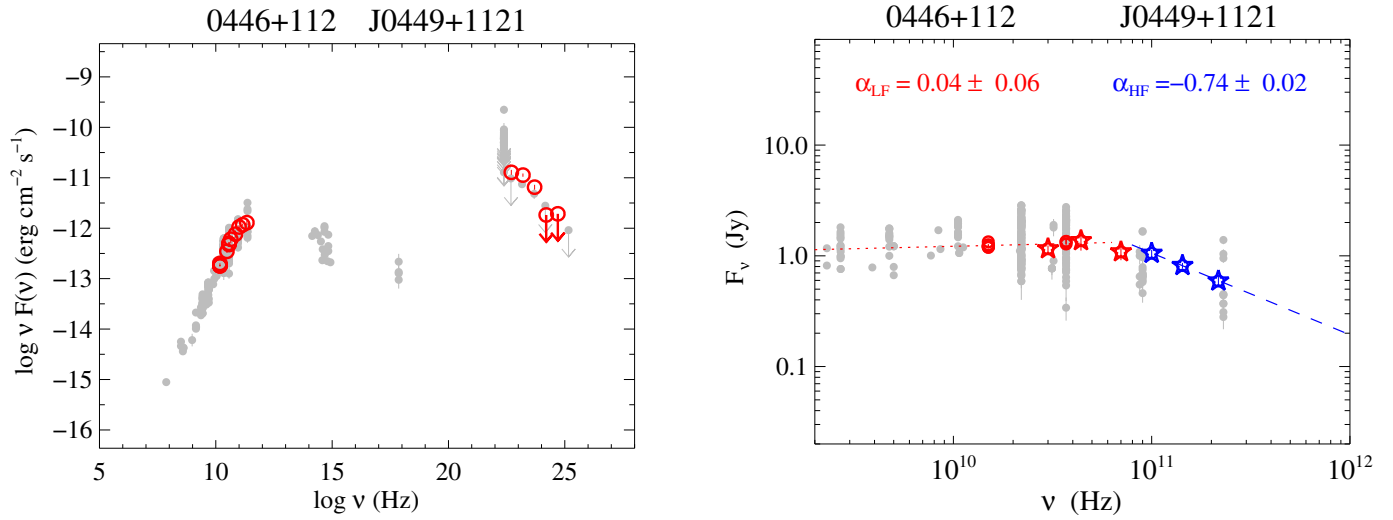
Fig. 40. 0446+112.
