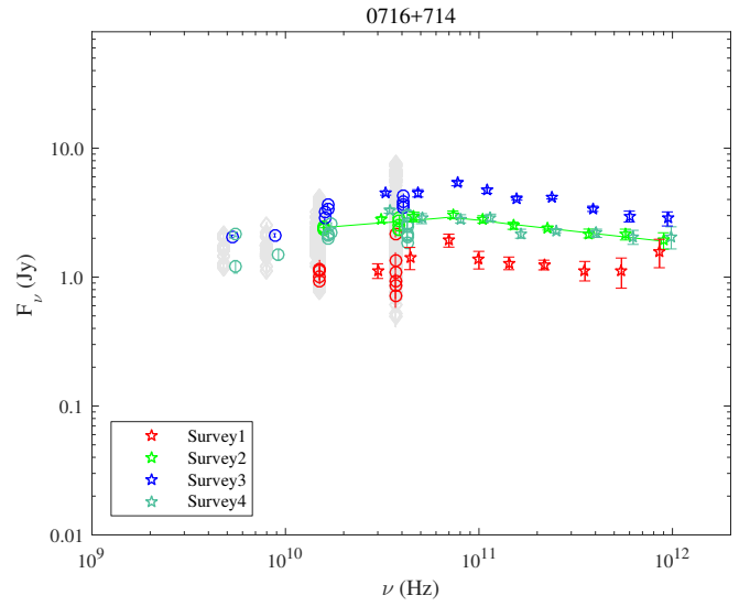
Fig. A.30. 0716+714.
