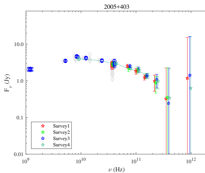
Fig. A.86. 2005+403.
