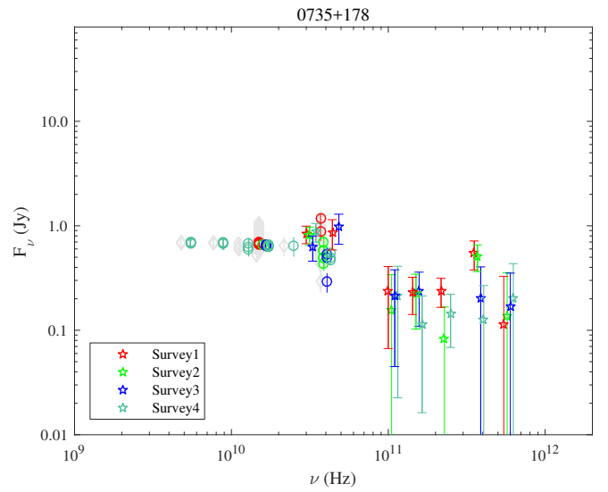
Fig. A.32. 0735+178.
