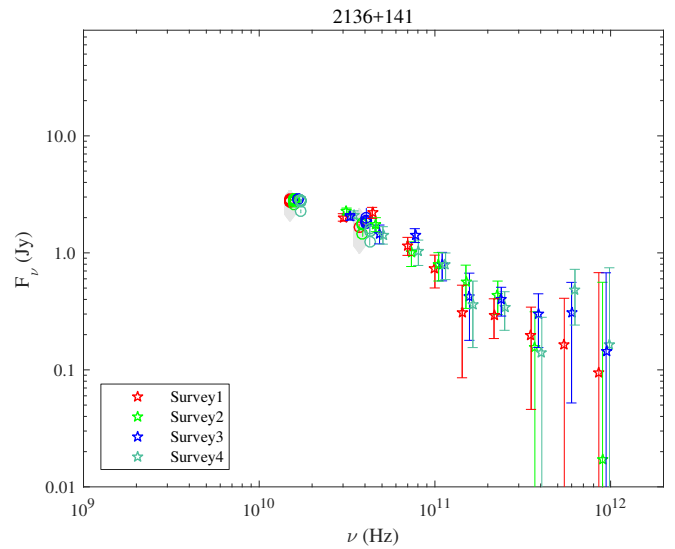
Fig. A.92. 2136+141.
