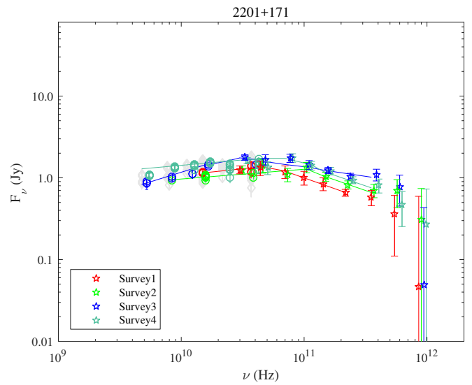
Fig. A.96. 2201+171.
