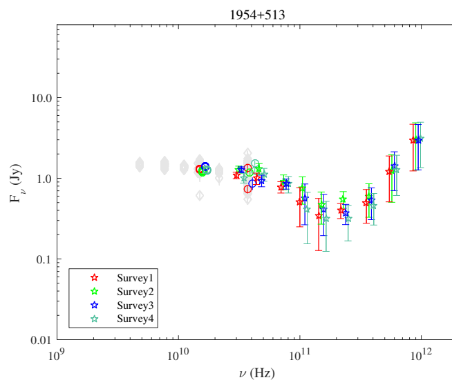
Fig. A.84. 1954+513.
