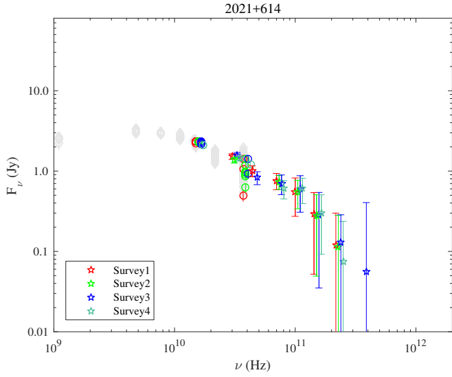
Fig. A.87. 2021+614.
