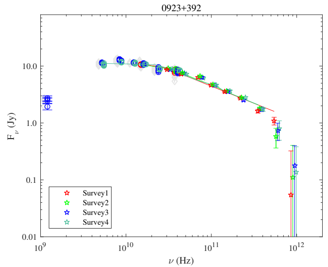
Fig. A.44. 0923+392.
