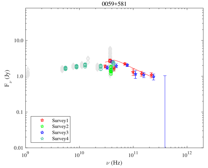
Fig. A.4. 0059+581.
