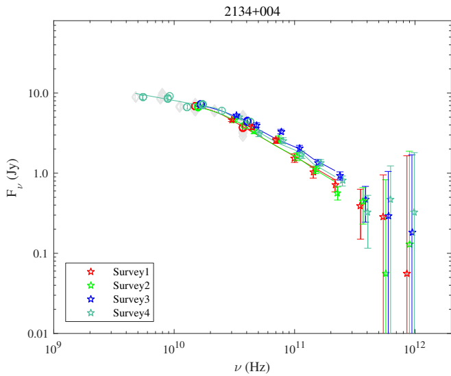
Fig. A.91. 2134+004.
