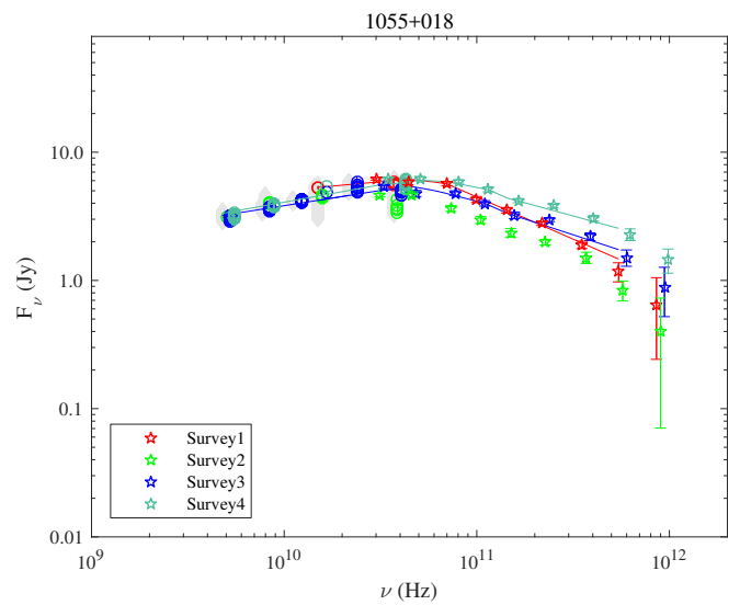
Fig. A.50. 1055+018.
