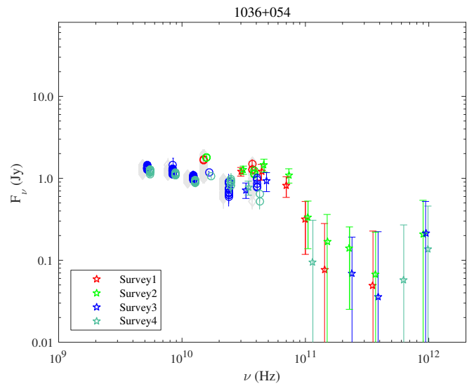
Fig. A.48. 1036+054.
