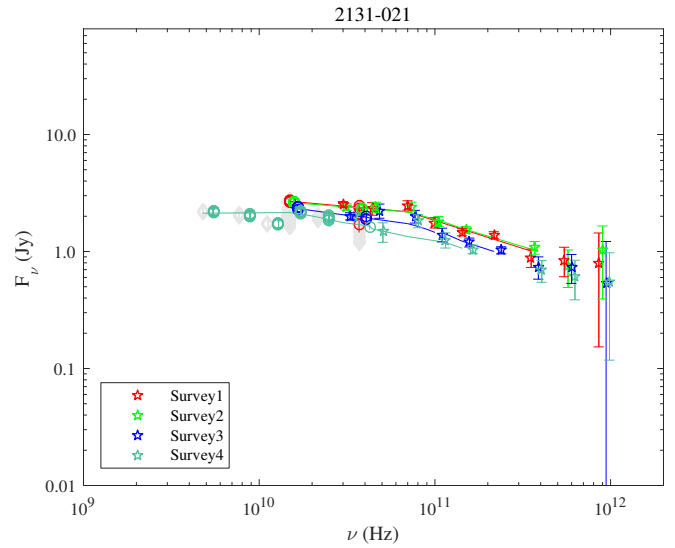
Fig. A.90. 2131-021.
