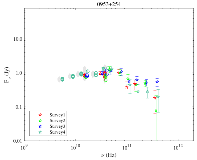
Fig. A.46. 0953+254.
