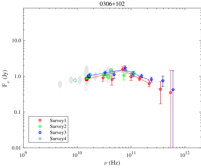
Fig. A.15. 0306+102.
