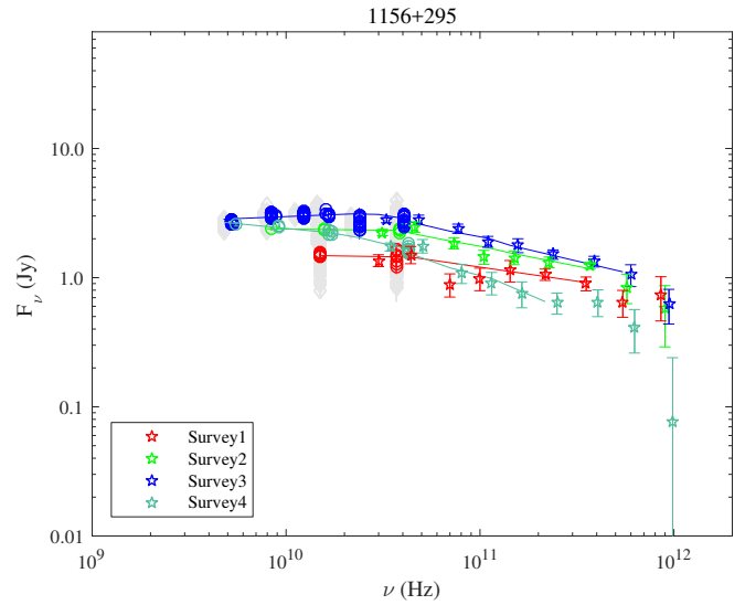
Fig. A.54. 1156+295.
