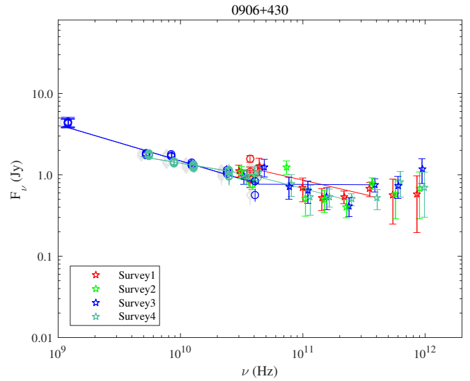
Fig. A.42. 0906+430.
