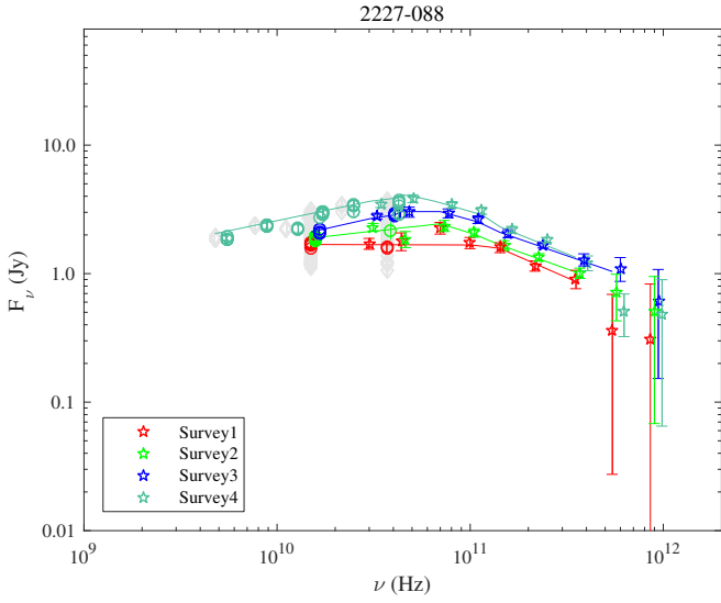
Fig. A.99. 2227-088.
