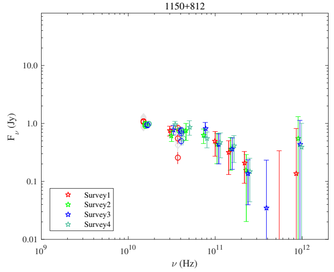
Fig. A.52. 1150+812.
