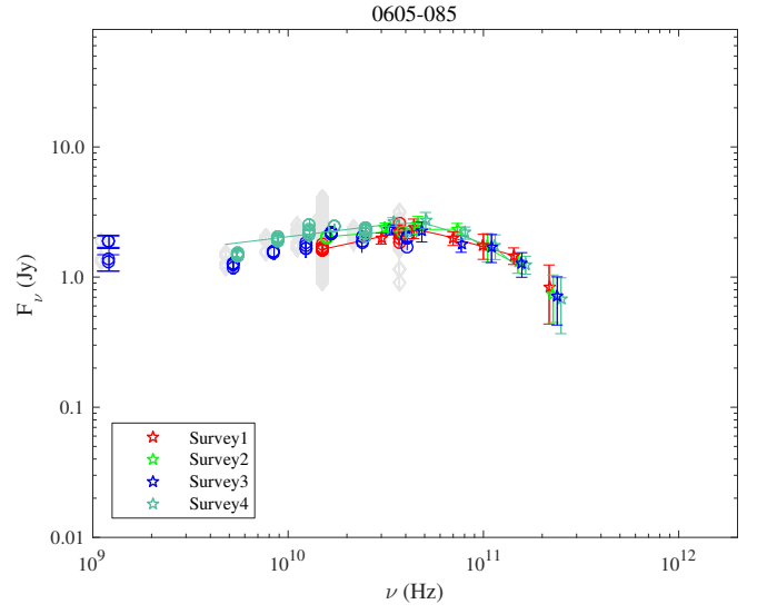
Fig. A.28. 0605-085.
