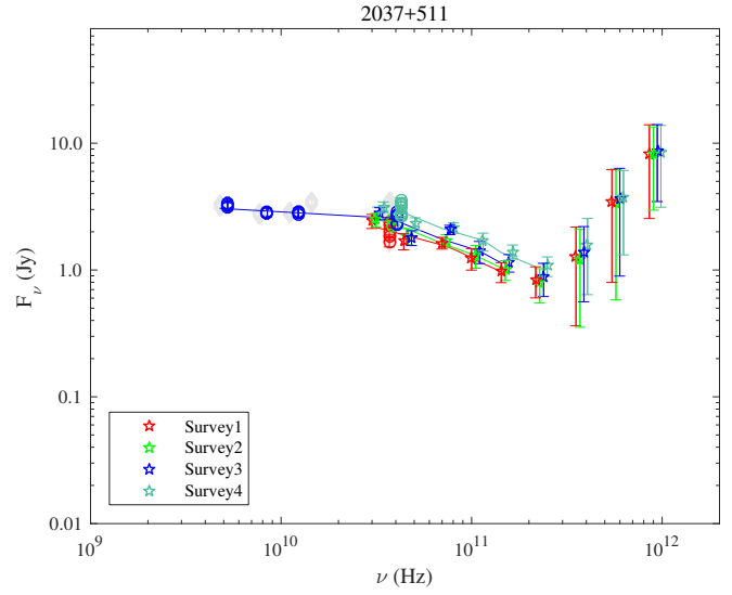
Fig. A.88. 2037+511.
