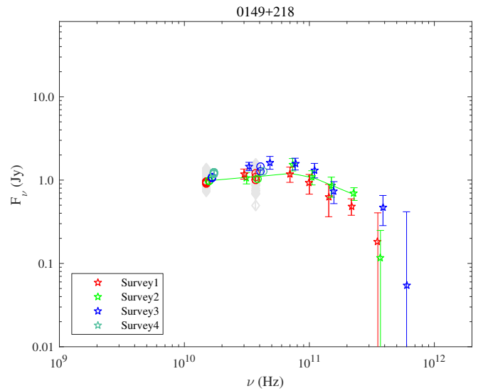
Fig. A.8. 0149+218.
