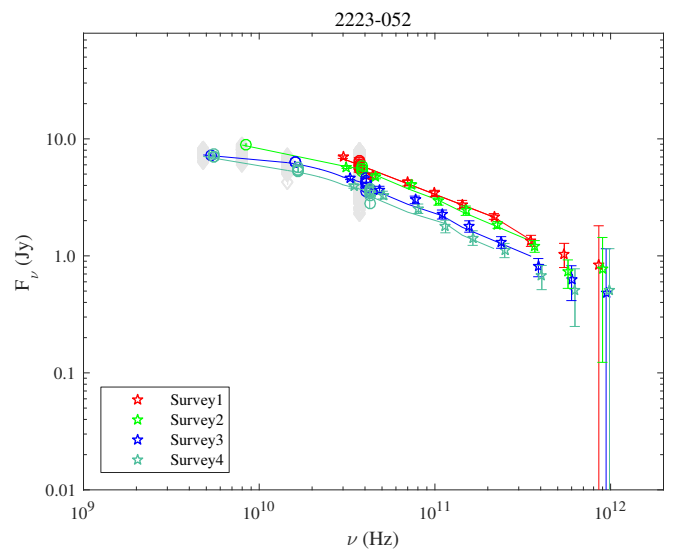
Fig. A.98. 2223-052.
