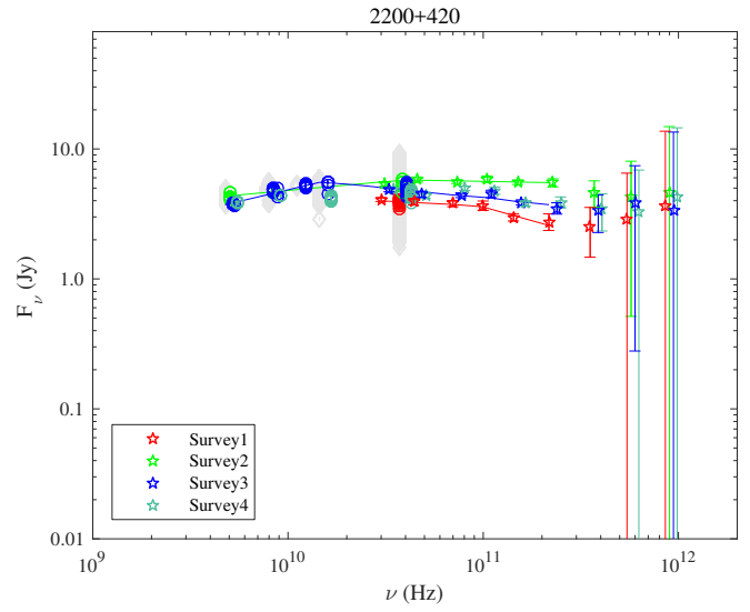
Fig. A.94. 2200+420.
