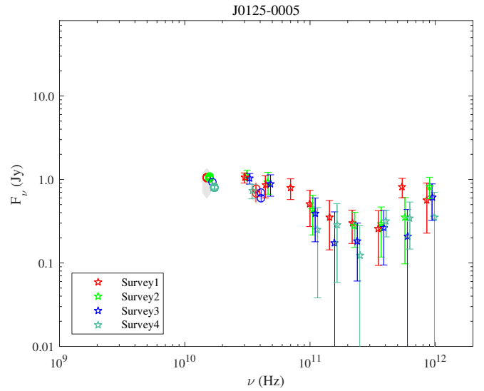
Fig. A.6. J0125-0005.
