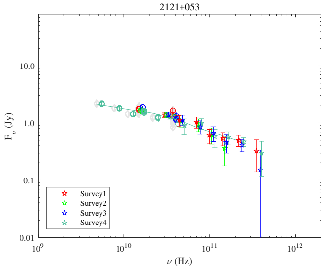
Fig. A.89. 2121+053.
