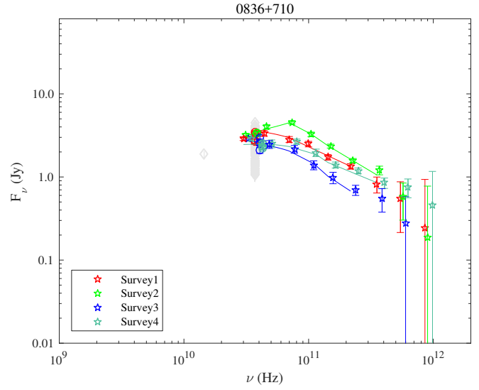
Fig. A.40. 0836+710.
