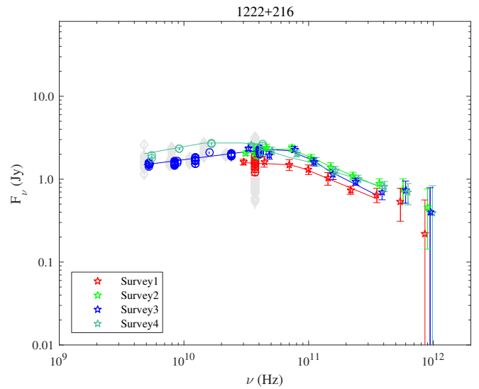
Fig. A.56. 1222+216.
