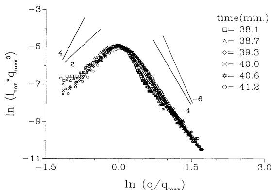
FIG. 4. \ln(I_{\text{nor}} q_{\text{max}}^3) vs \ln(q/q_{\text{max}}) .
