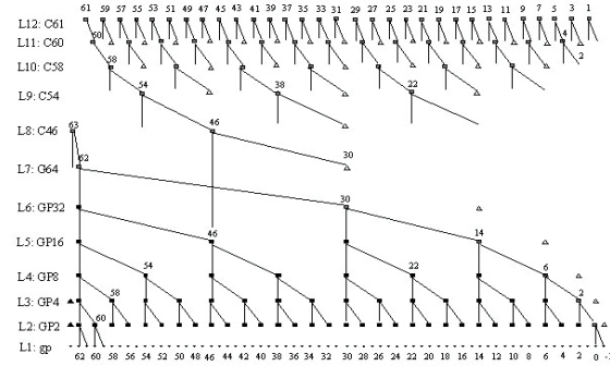
Fig. 9. Original Brent-Kung
