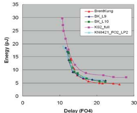
Fig. 17. Brent-Kung variants
