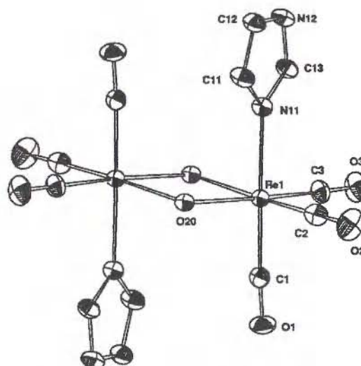
Fig. 3. ORTEP presentation of [Re 2 (im) 2 (μ-OH) 2 (CO) 6 ].
