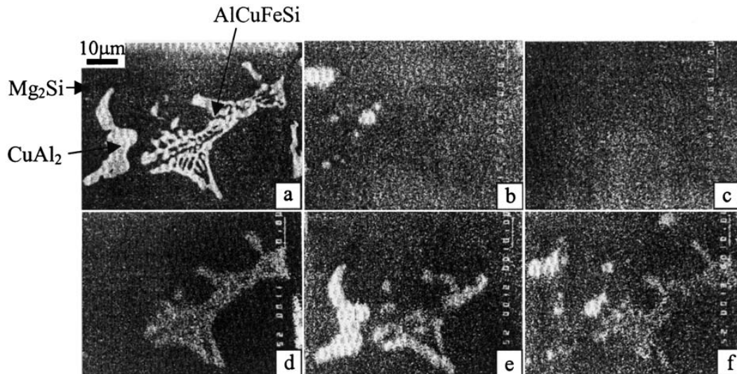
a BSE image; b Mg; c Mn; d Fe; e Cu; f Si
