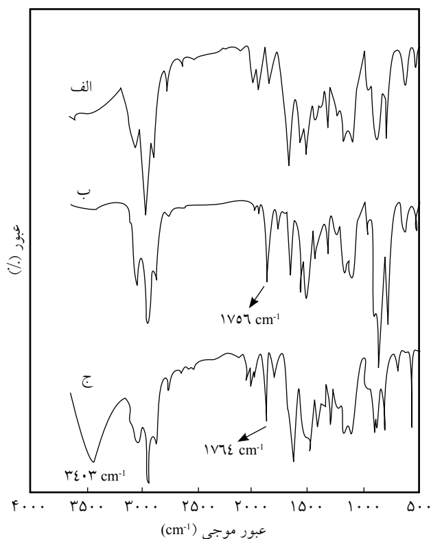
شکل ۴- طیف FTIR: (الف) کوپلیمر برم‌دار شده (استیرن- پارا متیل استیرن)، (ب) ترپلیمر متیل متاکریلات پیوند شده روی کوپلیمر (استیرن - پارا متیل استیرن) و (ج) نانوکامپوزیت پلیمری [PS/PMS)- g - PMMA]/Laponite RD.
