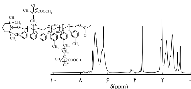
شکل ۵- طیف 1 H NMR ترپلیمر پیوندی پلی متیل متاکریلات روی کوپلیمر (استیرن- پارا متیل استیرن).
