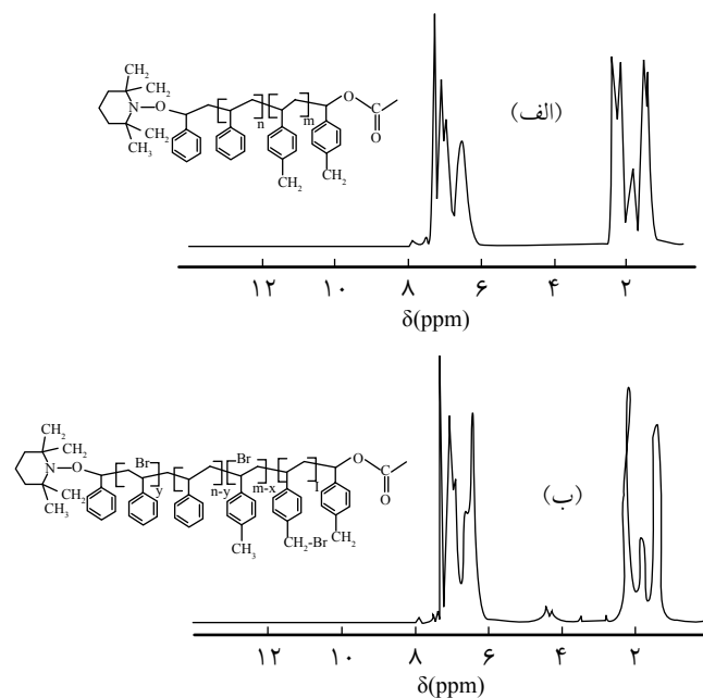
شکل ۳- طیف 1 H NMR: (الف) کوپلیمر (استیرن- پارا متیل استیرن) و (ب) کوپلیمر برم‌دار شده.
