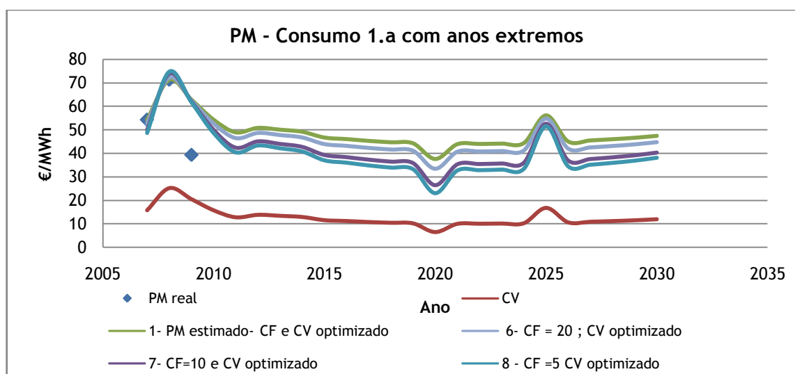
Figura 4.75 - Previsão Parcela de custos variáveis do total do sistema (CV) e Previsão do Preço do mercado (PM) até 2030 com as várias componentes fixas consideradas - Com inclusão de anos extremos.
