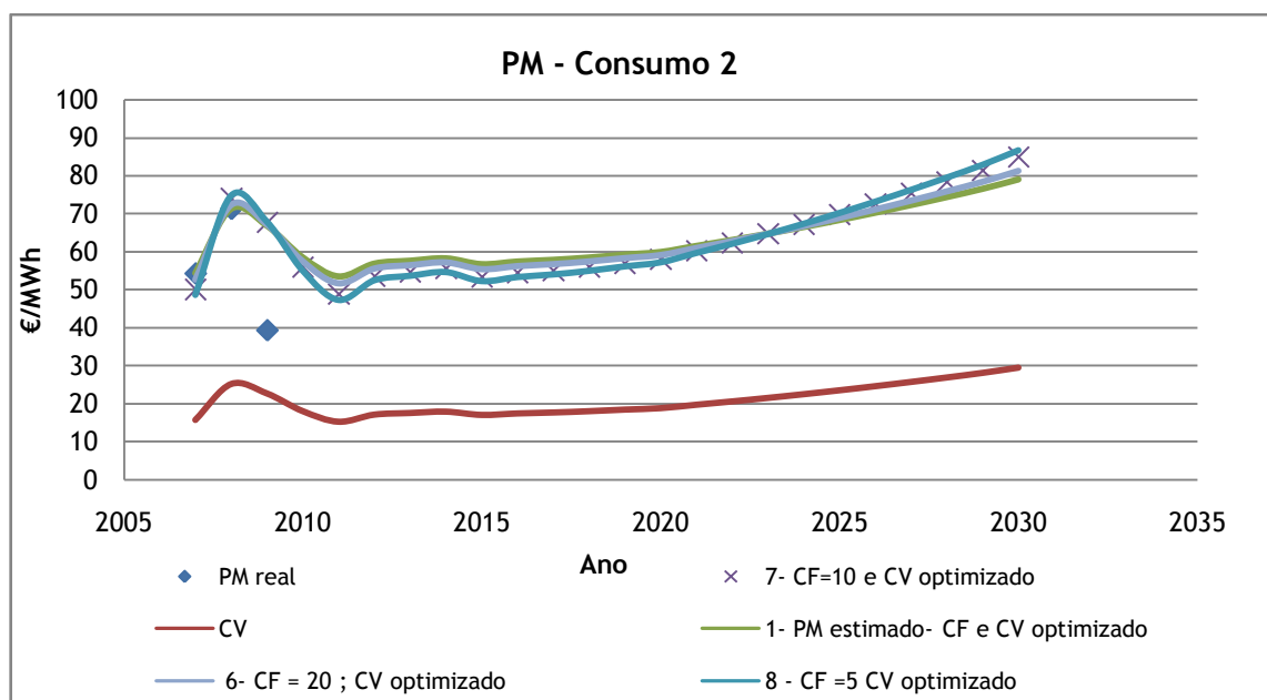
Figura 4.74 - Previsão Parcela de custos variáveis do total do sistema (CV) e Previsão do Preço do mercado (PM) até 2030 com as várias componentes fixas consideradas - Cenário P1 - Consumo 2
